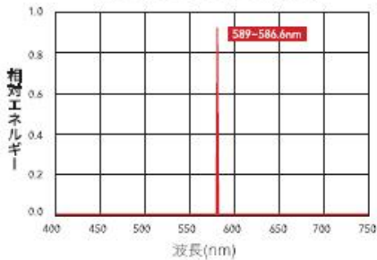
低圧ナトリウムランプの分光分布
